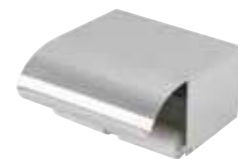
1005 Porta rotolo con coperchio Covered paper holder Porte rouleau avec couvercle Papierrollenhalter mit Deckel Бумагодержатель с крышкой cm 12 L x 13 P x 6 H
